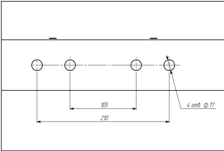
Рисунок 10.4 Монтажная площадка
