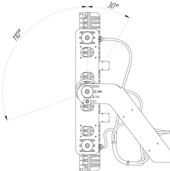
Рисунок 10.5 б. Установка прожектора на горизонтальную поверхность сверху. Предельные углы отклонения.
