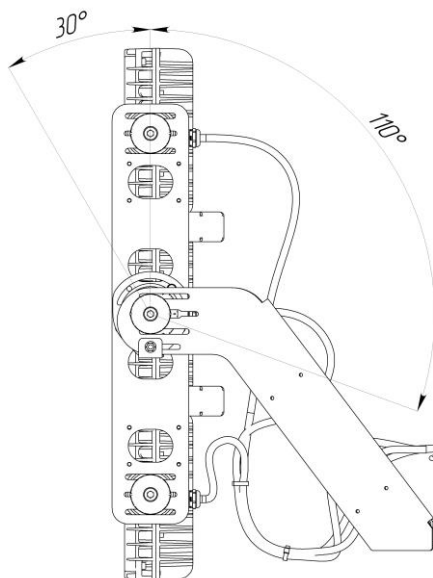
Рисунок 10.6 б. Установка прожектора на горизонтальную поверхность снизу. Предельный угол отклонения.
