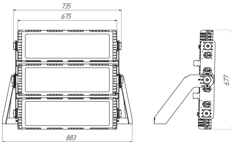
Рисунок 10.1 Габаритные размеры светильника
