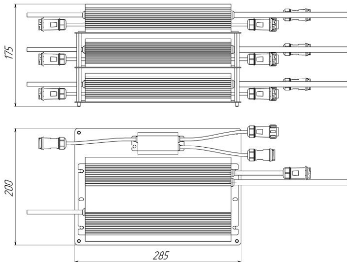
Рисунок 10.2 Габаритные размеры блока питания
