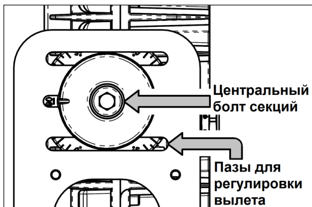
Рисунок 10.8 Регулировка вылета светодиодных секций
