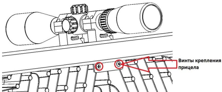
Рисунок 10.9 Крепление оптического прицела
