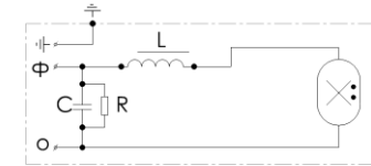
Рисунок 4 – Схема подключения к сети светильников РКУ21 «Гелиос»
