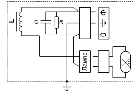
Рисунок 3 – Схема подключения к сети светильников РКУ21 «Гелиос»
