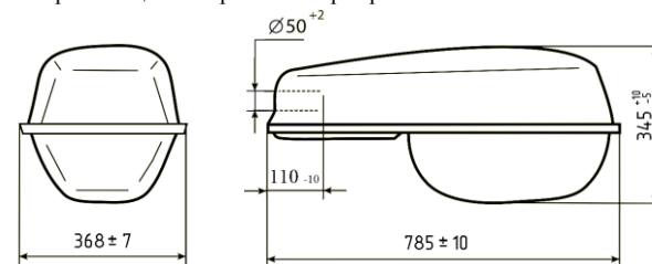
Рисунок 1 – Светильники серии ЖКУ15/РКУ15/ГКУ15...101/105/107
