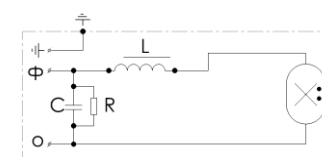
Рисунок 5 – Схема подключения к сети светильников РКУ15
