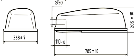
Рисунок 2 – Светильники серии ЖКУ15/РКУ15/ГКУ15...102
