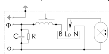
Рисунок 4 – Схема подключения к сети светильников ЖКУ15/ГКУ15
