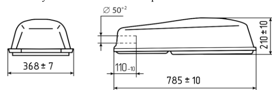
Рисунок 3 – Светильники серии ЖКУ15/РКУ15/ГКУ15...103
