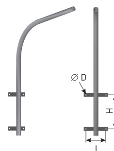
Рис. Б.4. — Характеристика установочных мест настенных кронштейнов (тип Н)
