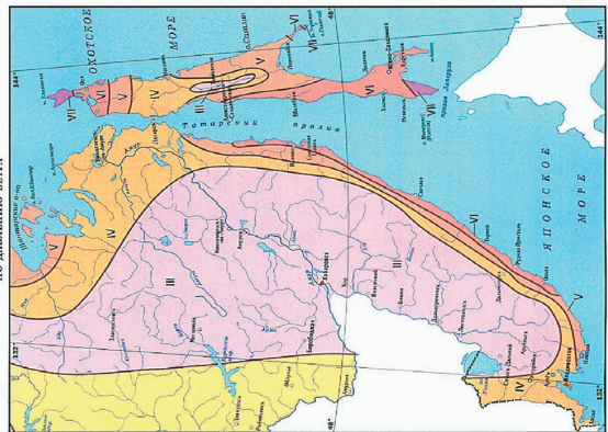
КАРТА 3в. РАЙОНИРОВАНИЕ ТЕРРИТОРИИ ПРИМОРСКОГО КРАЯ И ОСТРОВА СХЛИДИН ПО ДАВЛЕНИЮ ВЕТРА
