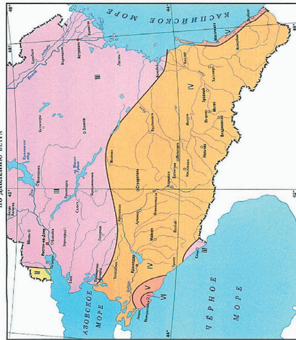
КАРТА 3к. РАЙОНИРОВАНИЕ ТЕРРИТОРИИ КАВКАЗА ПО ДАВЛЕНИЮ ВЕТРА
