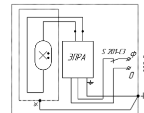
Рисунок 3 - Схема подключения к сети светильников с автоматическим выключателем
