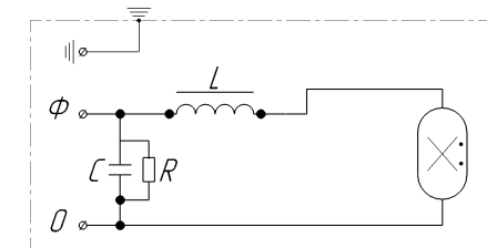
Рисунок 4 – схема подключения для РСУ24
