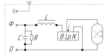
Рисунок 3 - схема подключения для ЖСУ/ГСУ24
