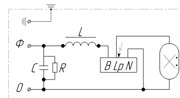
Рисунок 4 - схема подключения для ЖКУ/ГКУ24
