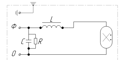
Рисунок 5 – схема подключения для РКУ24
